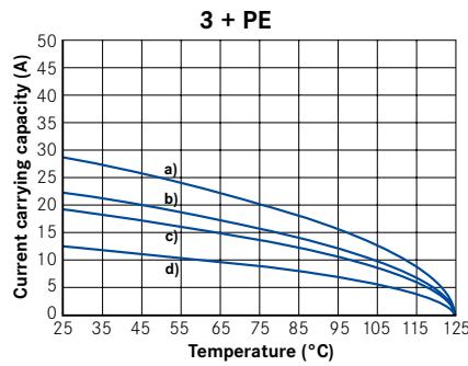
all contacts \varnothing 2,5 mm a) wire 4,0 mm 2 c) wire 1,5 mm 2 b) wire 2,5 mm 2 d) wire 0,5 mm 2
