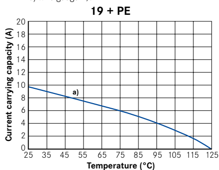
all contacts \varnothing 1,5 mm a) wire gauge 0,5 mm 2
