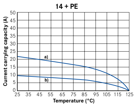
a) 4 contacts \varnothing 2,5 mm, wire gauge 1,5 mm 2 b) 11 contacts \varnothing 1,5 mm, wire gauge 0,5 mm 2
