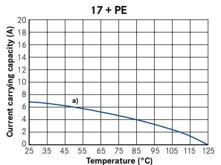
all contacts \varnothing 1,5 mm a) wire gauge 0,5 mm 2
