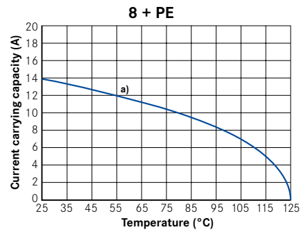
all contacts \varnothing 1,6 mm a) wire gauge 1,5 mm 2
